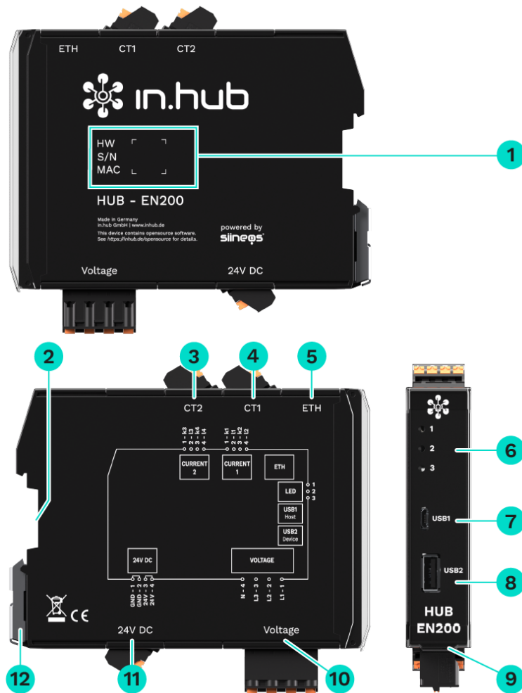
Ansichten des HUB-EN200 inkl. Schnittstellen
