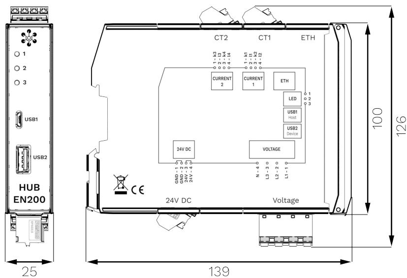
Abmaße des HUB-EN200 in mm
